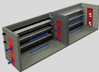
Kabelové kanály a kolektory vně objektu
